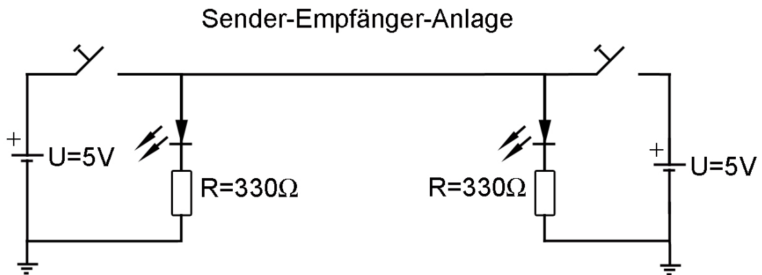
Abbildung 1: Morsetelegraf
